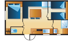
SUPER MERCURE 4/6 PERS 7,00 x 3,70 m - 25,7 m 2
